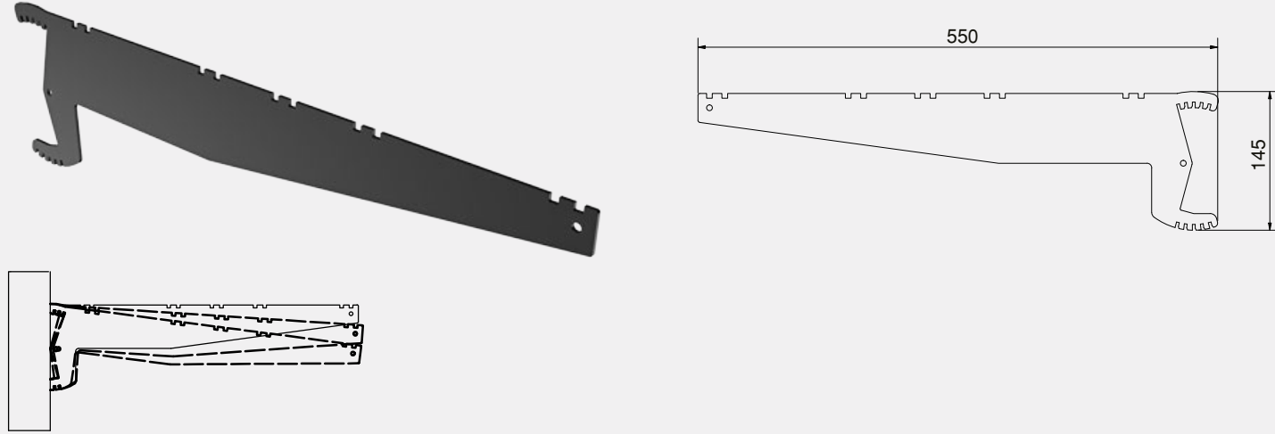
550 KONSOL 550 CONSOLE
